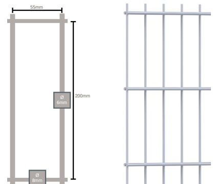
Maille du panneau KOLOSS® 868 Premium
