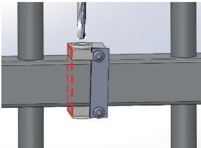
L'outil facilite les opérations : le perçage est guidé et la découpe des lisses est parfaitement droite.
