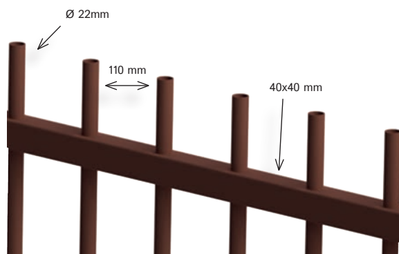
Barreaudage Tivano® couleur : Corten (Classe 1)
